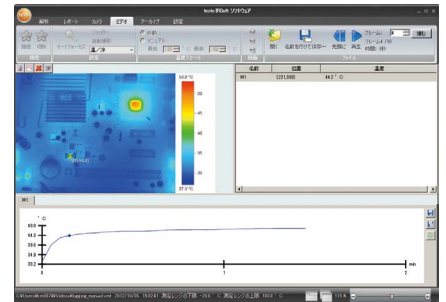
最大15のマーカーをつけられ、各ポイントの トレンドグラフを表示
